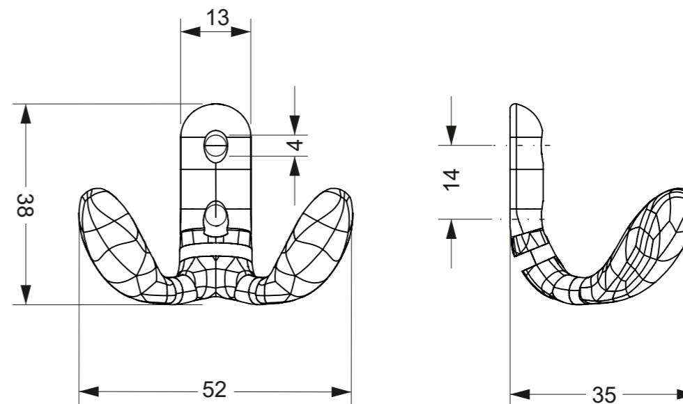
704 GANCIO COLIBRI MODELLO DOPPIO TIPO PICCOLO
