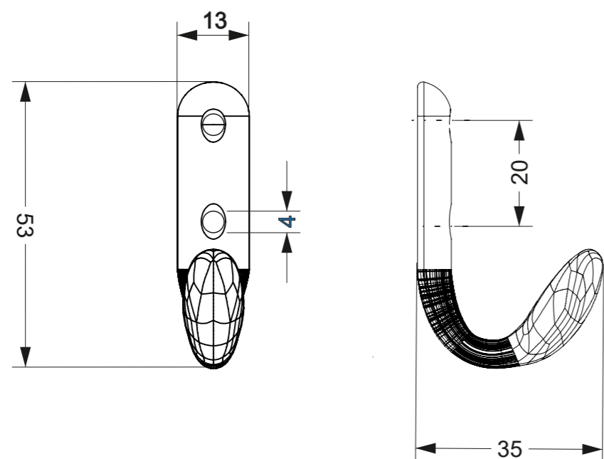
705 GANCIO COLIBRI MODELLO SINGOLO TIPO GRANDE
