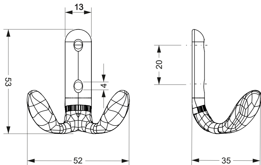
703 GANCIO COLIBRI MODELLO DOPPIO TIPO GRANDE
